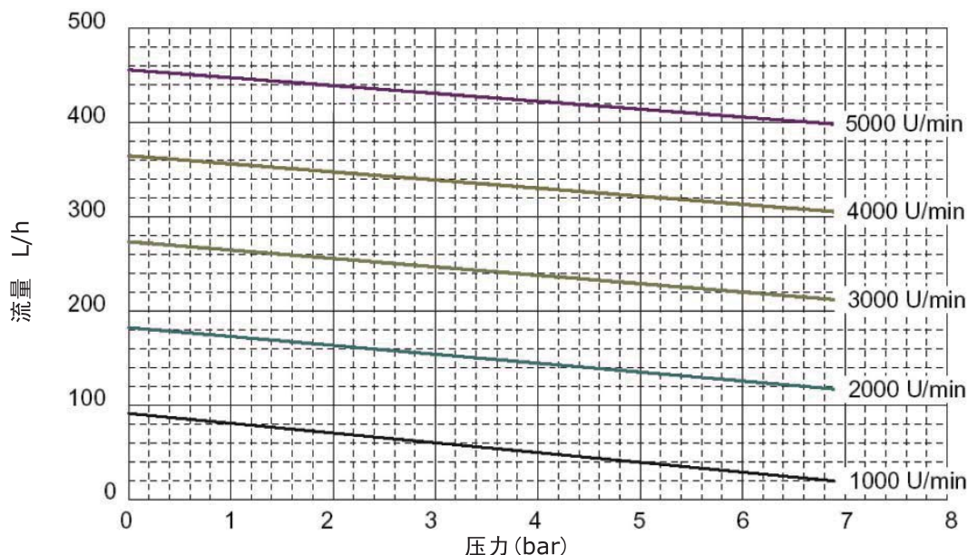
技术曲线图
