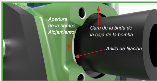
Figura 10 Anillo de Fijación de Dura 10, 15, 25 y 35 Insertado
