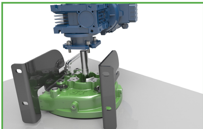
Figura 5 Instalación de la Unidad del Motor con Reductor
