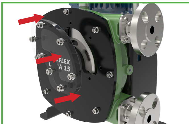
Figura 13 Colocación de la Ventana de Inspección
