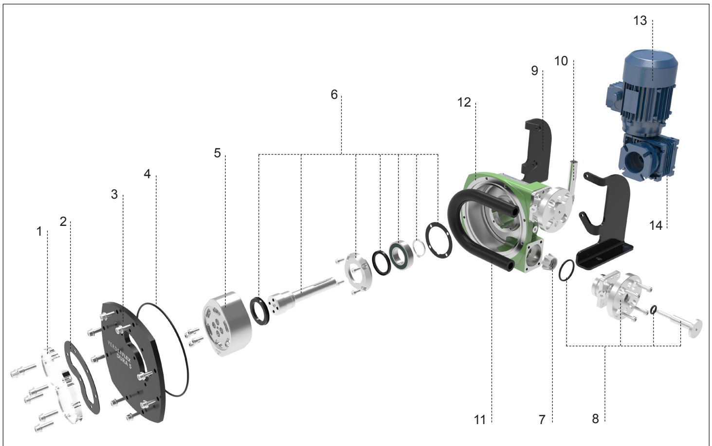
Figure 3 Vista Desarrollada de Dura MK IV 5 y 7 (Vista Genérica)
