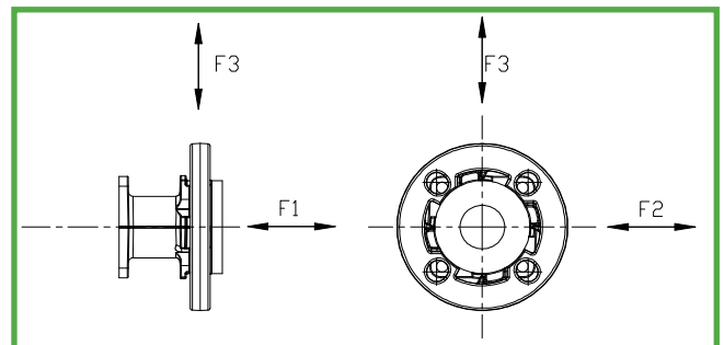
Figura 14 Cargas de la Boquilla en las Bridas
